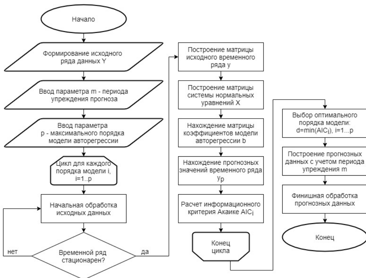
Рис.3. Блок-схема алгоритма прогнозирования доходов МО с использованием модели авторегрессии
